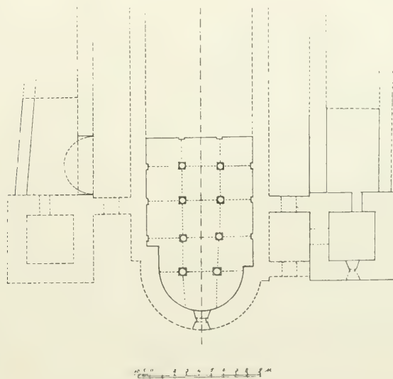
Fig. 51. Rekonstrukcja planu zachodniej części kościoła romańskiego.
